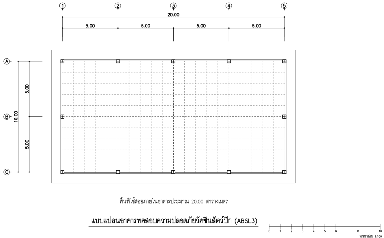
รูปที่ 10 แสดง Conceptual layout ของอาคารทดสอบความปลอดภัยวัคซีนสัตว์ปีกของโครงร่างเดิม
